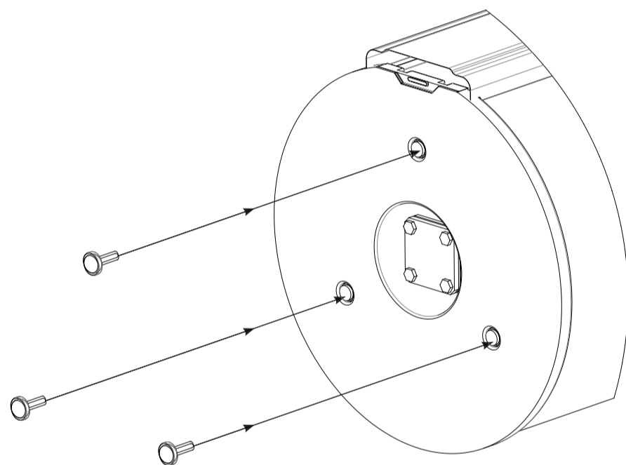
Montage der Stellfüße
